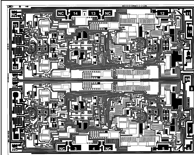
INA2141 DIE TOPOGRAPHY
